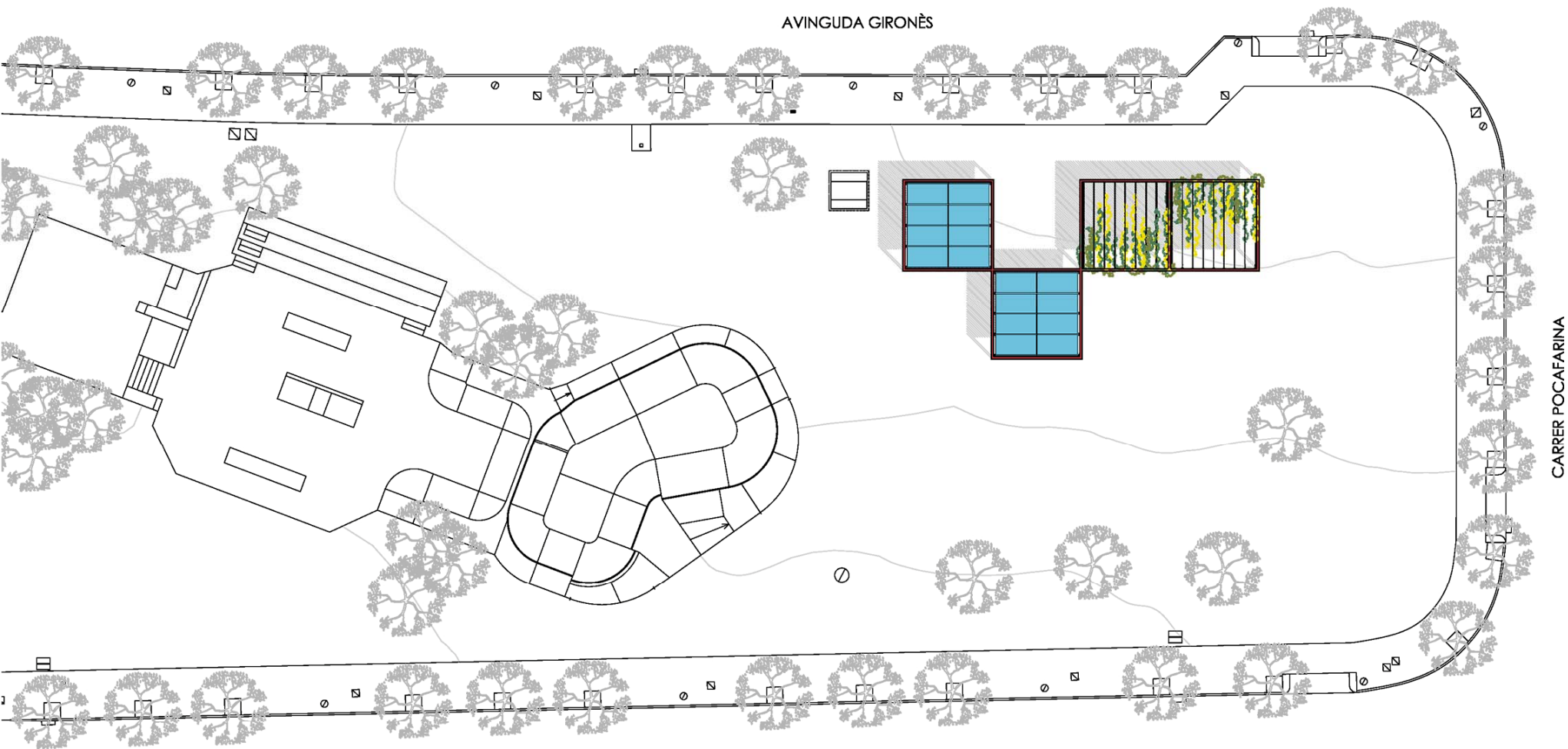
pèrgola a Skatepark, Llagostera emplaçament: Av. del Gironès 51 i Av. de l'esport
