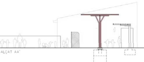
pèrgola al CEIP Dr. Sobrequès. emplaçament: Plaça de les Nacions 8. Bescanó
