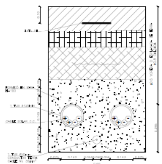
SECCIO 2. RASA ENTRE ARQUETES, 2ºEPI25 ESC 1:15
